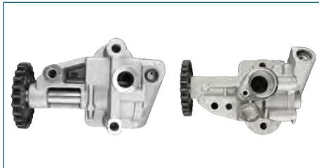
BOMBA ACEITE 07K115105Q
