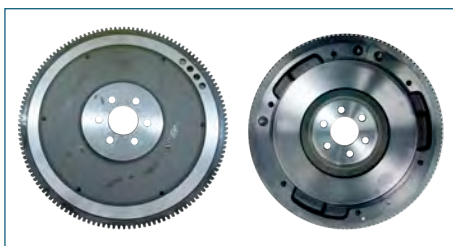
VOLANTE MOTOR 93382757
