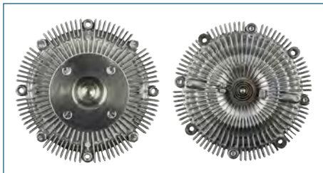
FAN CLUTCH 21082VB100 FAN CLUTCH D22 (2002-2008) 2.5DIESEL - URVAN (2013-2018) 2.5DIESEL
