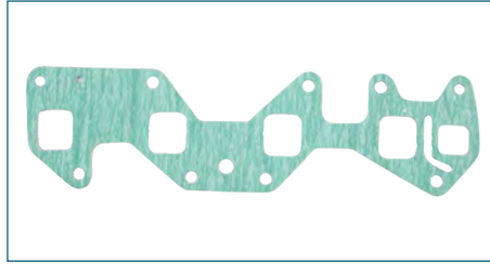
JUNTA MULTIPLE 90323399
