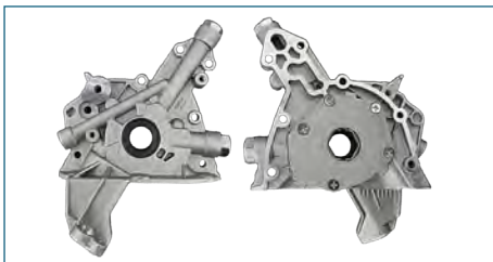
BOMBA ACEITE 93377141
